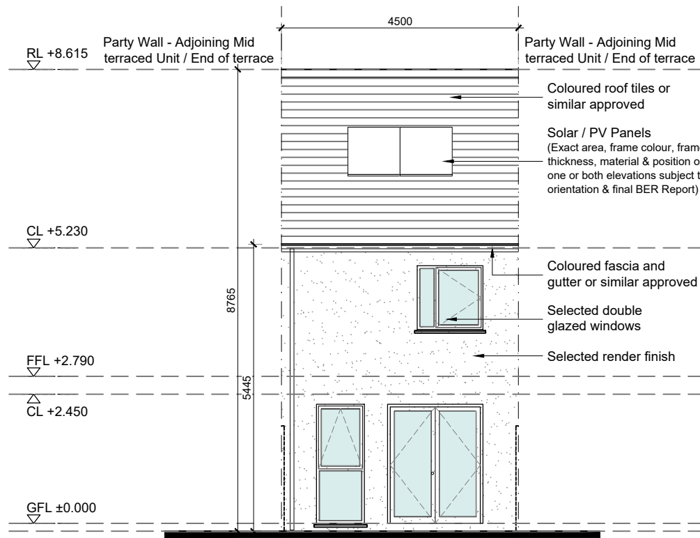
02 Rear Elevation 1:100 @ A3
